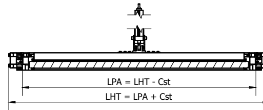
A-A ( 1:10 )
