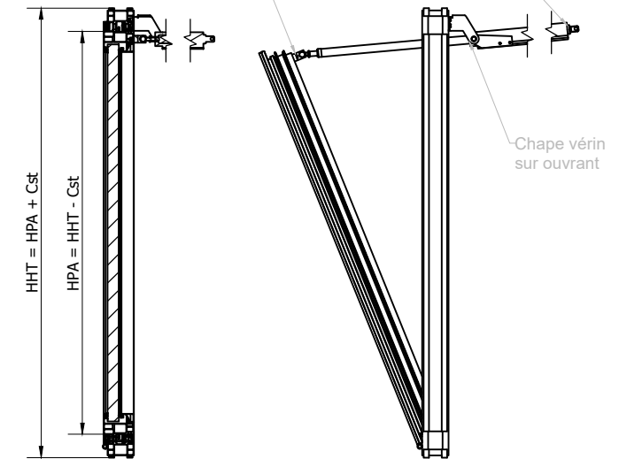
B-B ( 1:10 )
